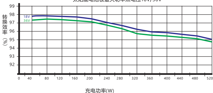
12V系统转换效率曲线 太阳能电池板最大功率点电压18V/36V
