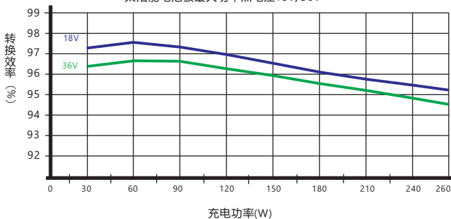
12V系统转换效率曲线 太阳能电池板最大功率点电压18V/36V
